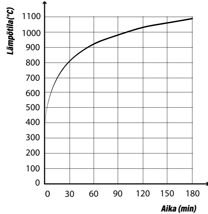
Standardien ISO 834-1 ja EN 1363-1 mukainen testiympäristön lämpötilakäyrä.
